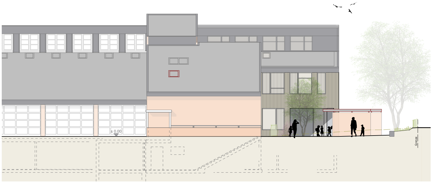
Ansicht West
