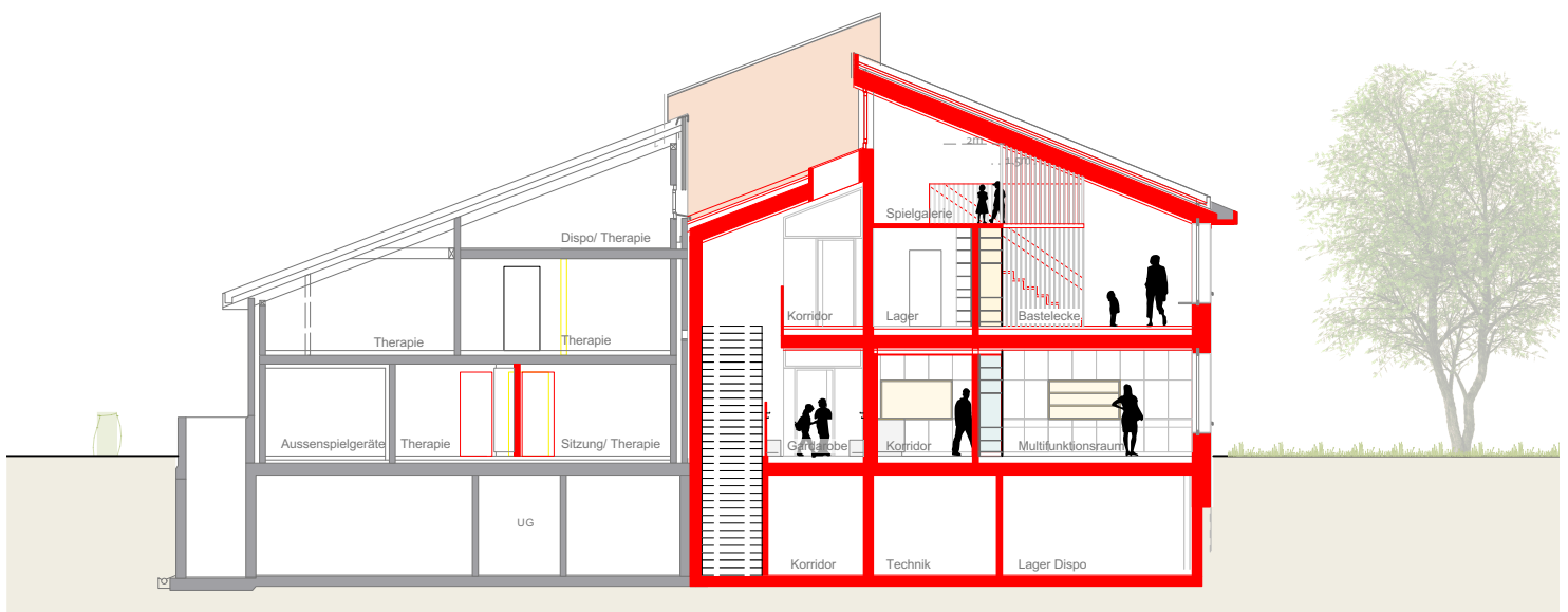
Querschnitt
