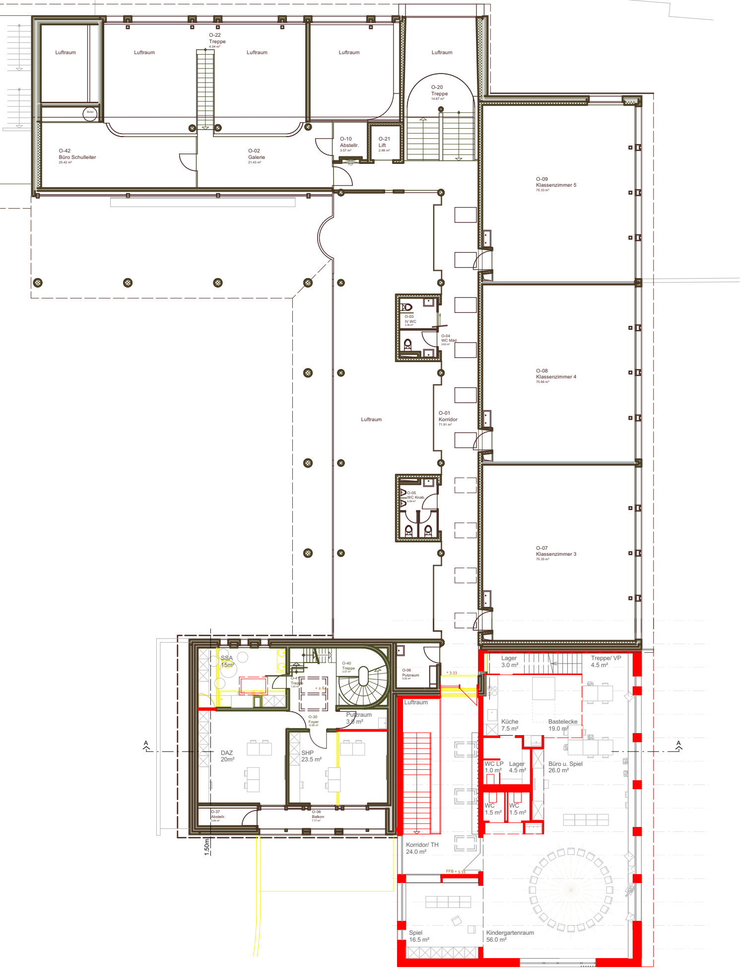
Obergeschoss
